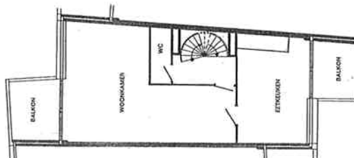
B3 WOONVERDIEPING
