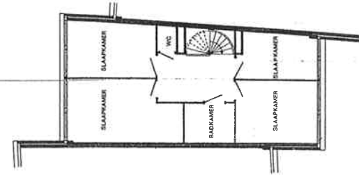
C4 SLAAPVERDIEPING
