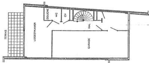
A2 PARTERRE
